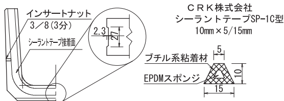
目地部詳細図
