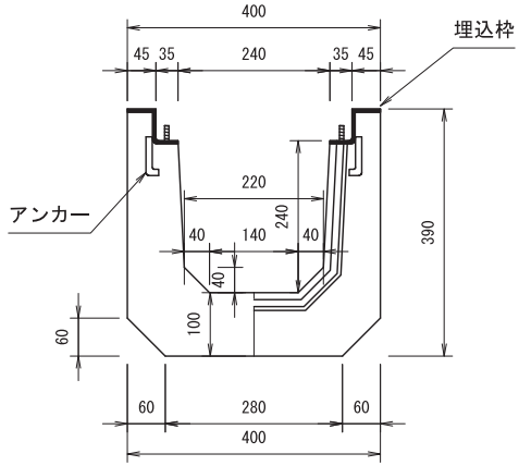
横断側溝GT-240
