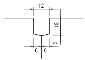
目地詳細
