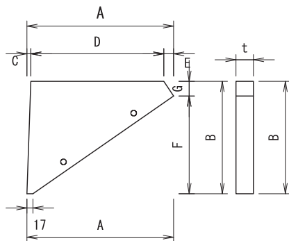
連結仕様 W 1/2 L=75mmボルト n4
