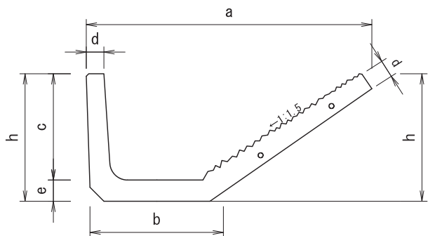
寸法図
