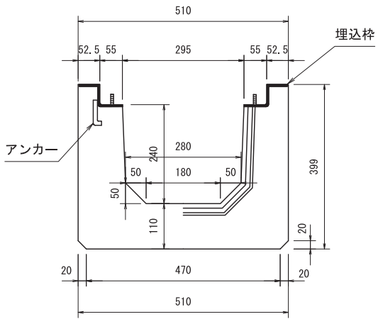
横断側溝GT-300B
