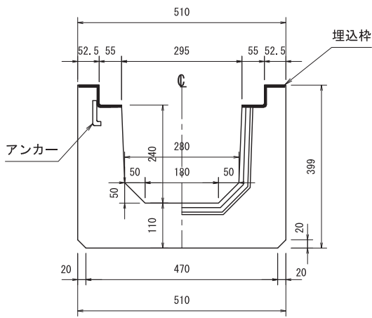
横断側溝GT-300A
