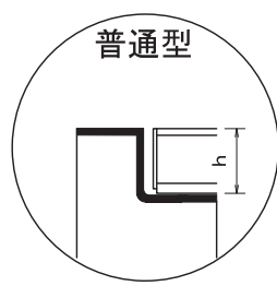
横断側溝GT-240
