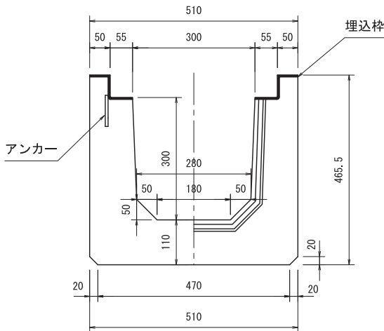
横断側溝GT-300B
