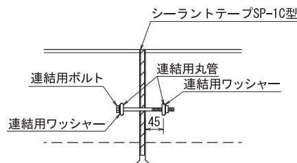
連結部詳細図
