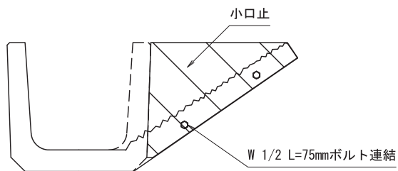
施工略図
