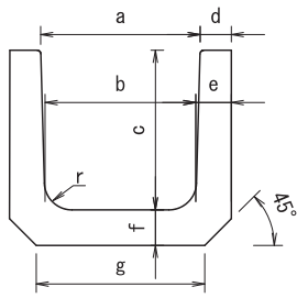
呼び名 U-180以下
