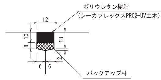
止水用目地詳細
